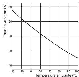
G3NA-2□□B-UTU entrée c.a.
